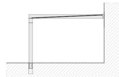
DOORSNEDE ULTRALINE COMPACT
