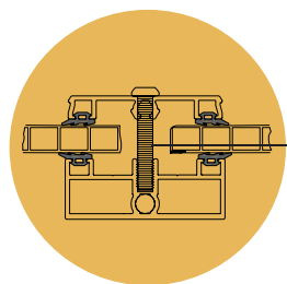
Bevestiging van twee polycarbonaat platen.
