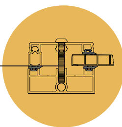
Bevestiging van polycarbonaat in een zijsluitprofiel.
