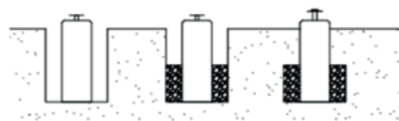
Zijaanzicht plaatsing betonpoer.
