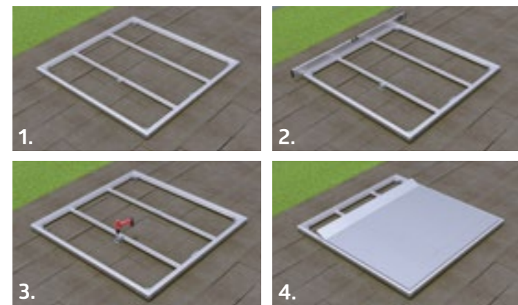
1. Montage van het frame 3. Schroef de stelvoeten vast 2. Stelvoeten bevestigen en het frame uitlijnen 4. Alu-platen verleggen en bevestigen
